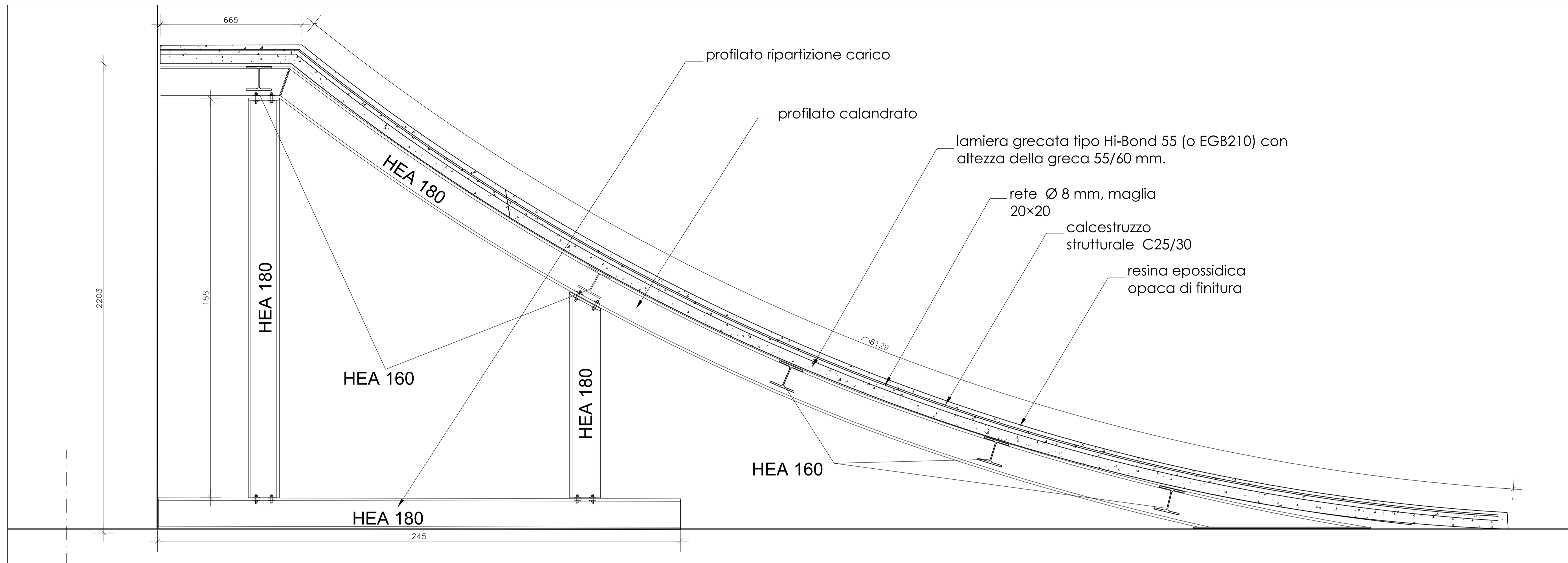
SEZIONE A-
