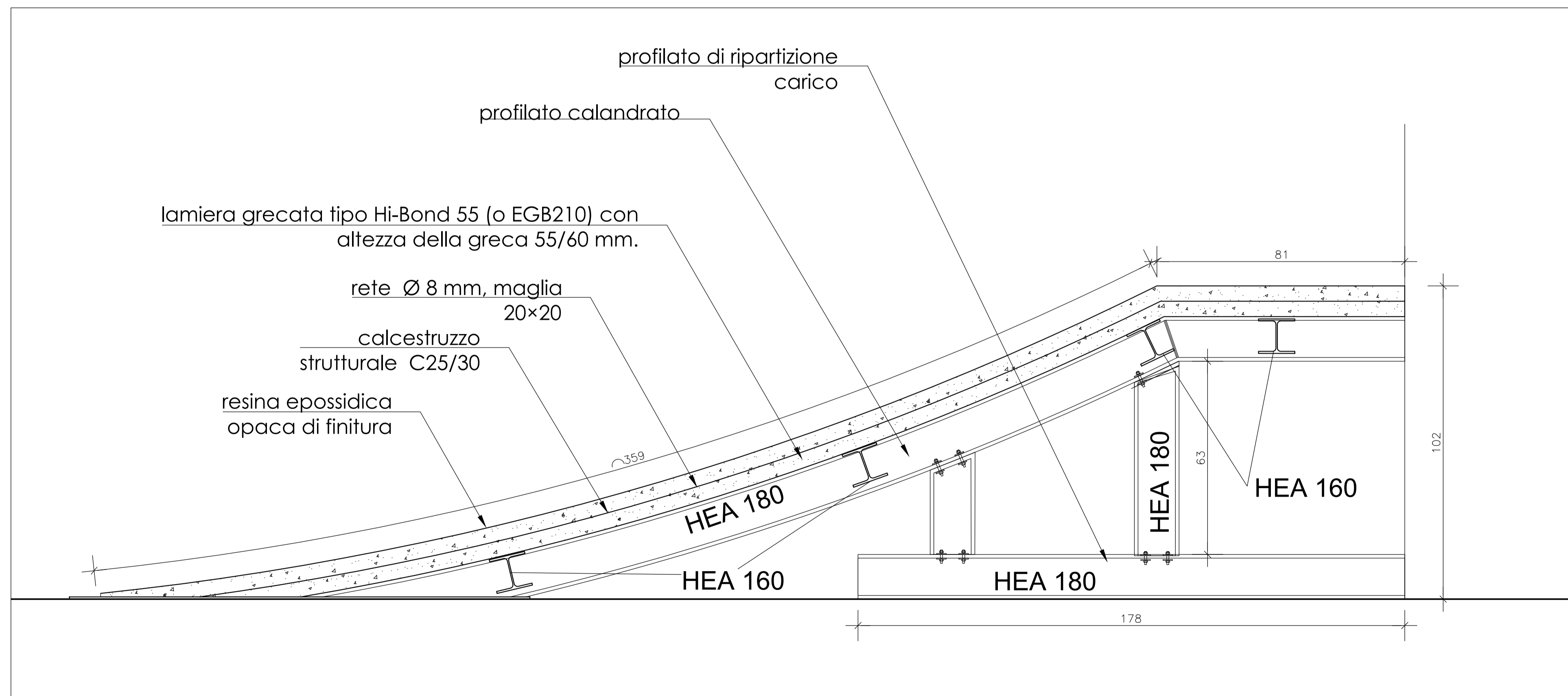
SEZIONE B
